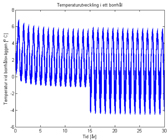
Figur 19: Borrhållslängd 70m. Borrhålets väggtemperatur.
