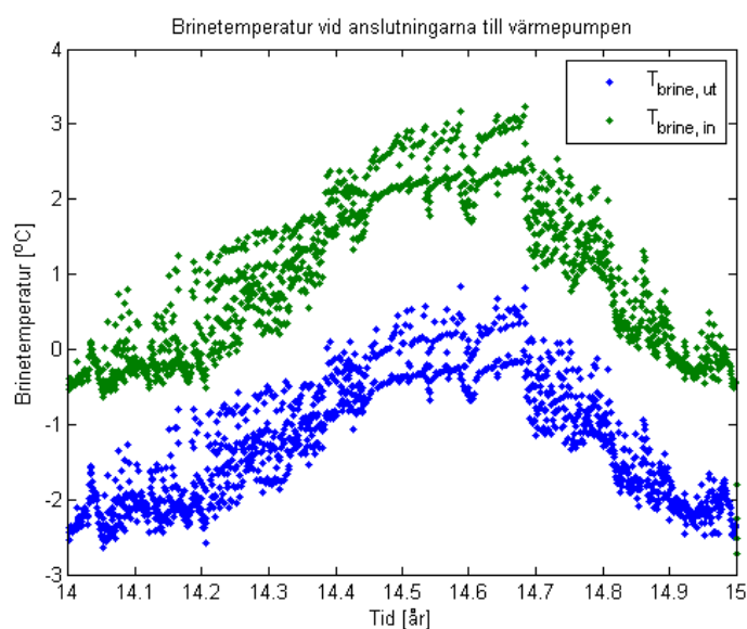
Figur 26: Brinetemperaturer i värmepumpen, 100 m enskilt hål, gammal värmepump.
